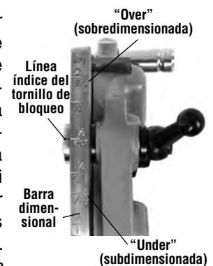
Figura 11 – Ajuste del tamaño de la rosca
