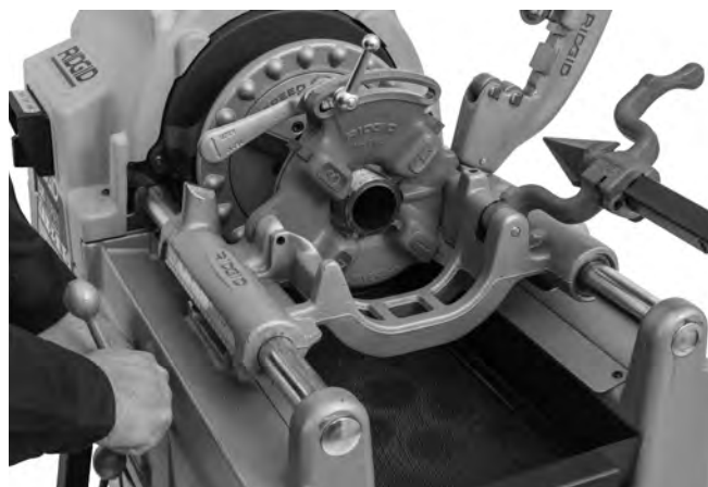
Figura 23 – Roscado de un tubo
