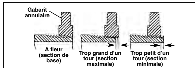
Figure 27 – Contrôle de la section du filetage
