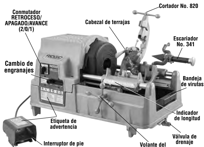
Figura 2A – Roscadora de mandril automático 535
